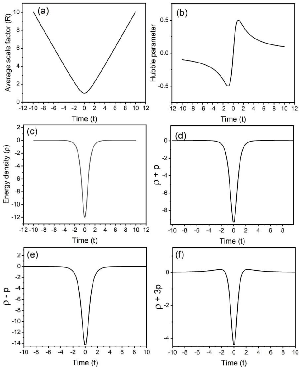
Fig. 1 Plots of time versus (a) Average scale factor (b) Hubble parameter (c ) Energy density ( \rho ) (d) \rho + p (e) \rho - p (f) \rho + 3p
